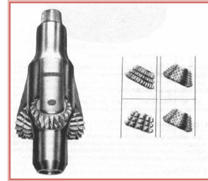
Kılavuzlu genişleticiler
