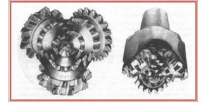
Üç çeneli matkap (Sert, kaya formasyonlarda)
